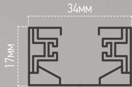
СЕЧЕНИЕ ШИНОПРОВОДА СЕРИИ SB
