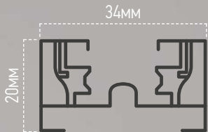
СЕЧЕНИЕ ШИНОПРОВОДА СЕРИИ RB
