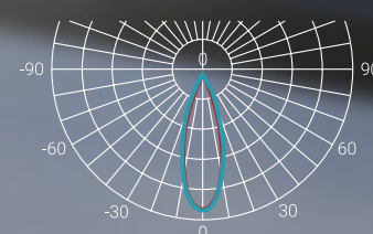
Кривая силы света (КСС) – К
