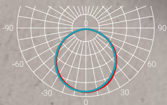
Кривая силы света (КСС) – Д
